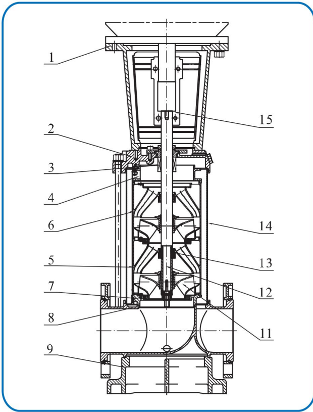
截面图 CDL,CDLF120,150,200
